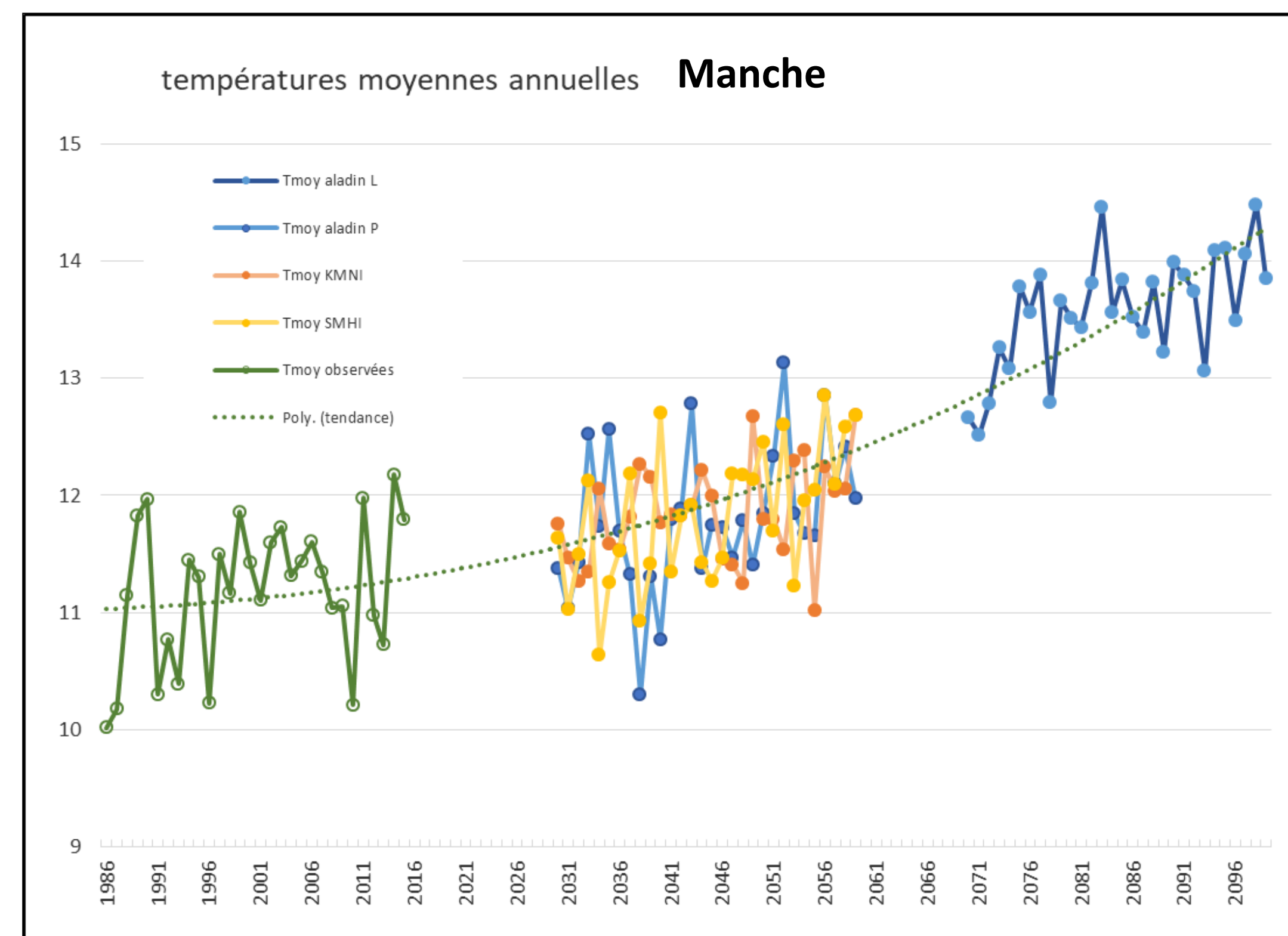
Evolution des températures moyennes annuelles, de 1986 à 2096
