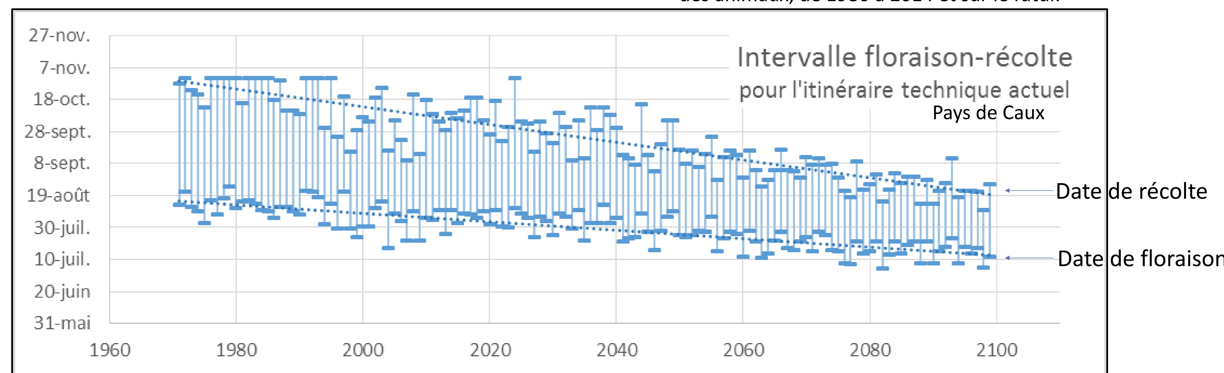
Evolution des dates de floraison et récolte du maïs pour la combinaison précocité x date de semis actuelle
